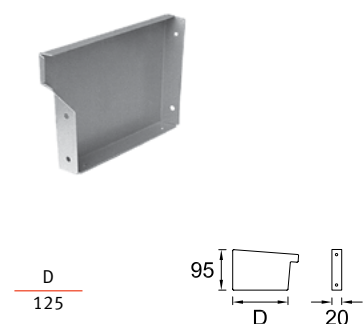
354 Заглушка ринви ліва
