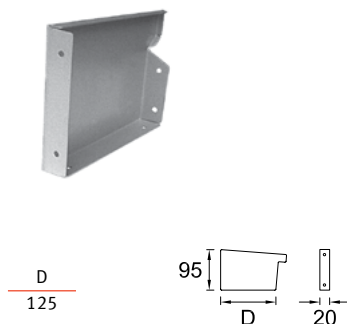
353 Заглушка ринви права
