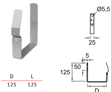
345 Кронштейн ринви довгий
