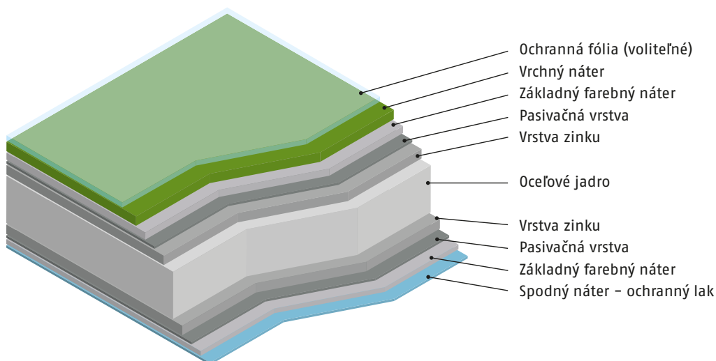
Prierez plechu
