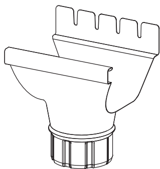
Apaļš notekcaurules konektors
