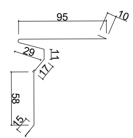
2. Rästyslista taittuva, pystysaumakatteet, L = 3000 mm
