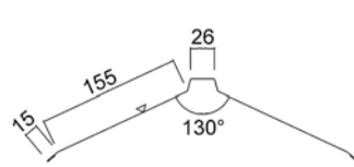
2. Harjalista sileä, L = 3000 mm
