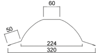
2. Harjalista pyöreä, L = 2100 mm
