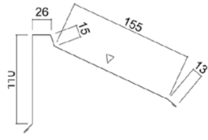
9. Pulpettikaton ylärästyslista, L = 3000 mm
