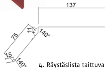
4. Räystäslista taittuva, teräskatteet, L = 3000 mm
