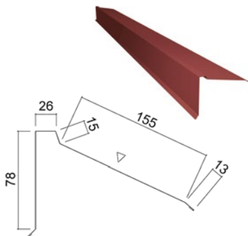
Pulpettikaton yläräystäslista, L = 3000 mm
