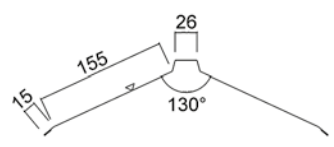
4. Harjalista sileä, L = 30000 mm
