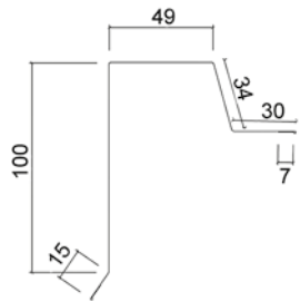
1. Päätylista, pystysaumakatteet, L = 3000 mm
