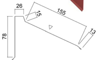
Pulpettikaton yläräystäslista, L = 3000 mm
