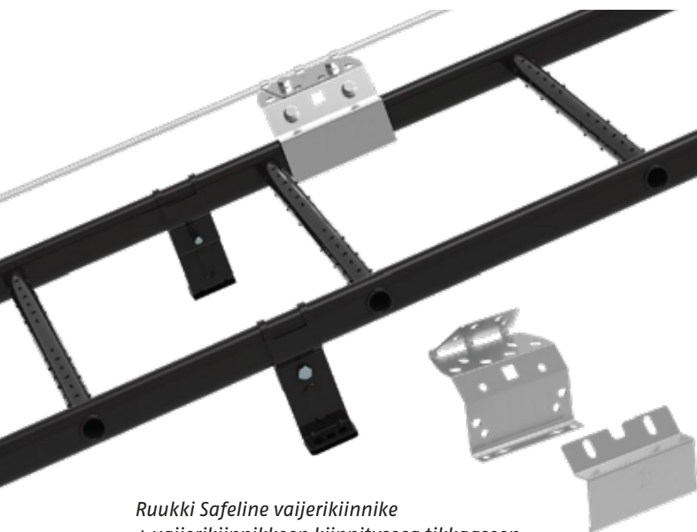
Ruukki Safeline vaijerikiinnike + vaijerikiinnikkeen kiinnitysosa tikkaaseen + liukukiinnikkeen avattava pysäytin tikkaaseen
