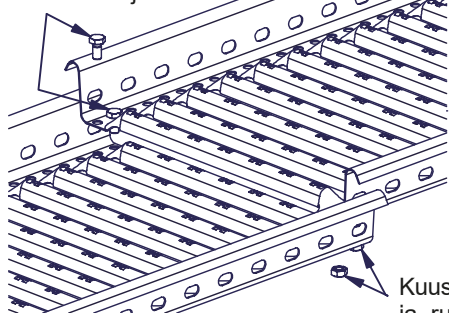
Kuusiomutteri ja -ruuvi
