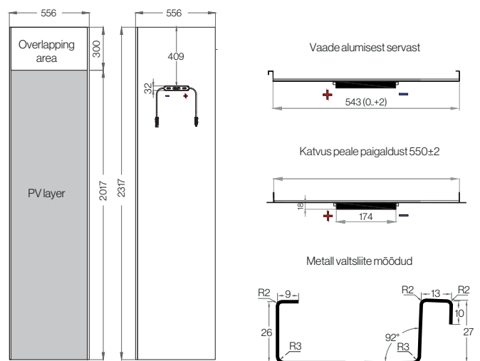
Tehnilised joonised (mm)
