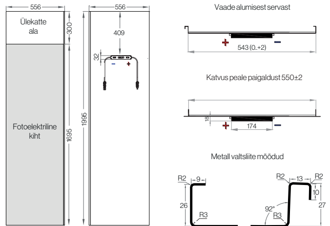
Tehnilised joonised (mm)
