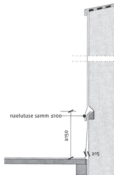
Joon. 54 Tulemüür. Mastaap 1:10
