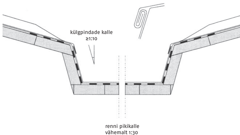
Joon. 26 Renni alla pannakse hüdroisolatsioonikiht.
