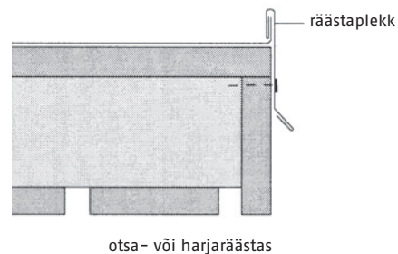
Joon. 47 Räästaplekk naelutatakse maksi- maalselt 800 mm sammuga. Mastaap 1:5
