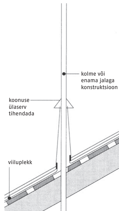
Joon. 53 Jäiga konstruktsiooni läbiviigu koonus. Mastaap 1:10
