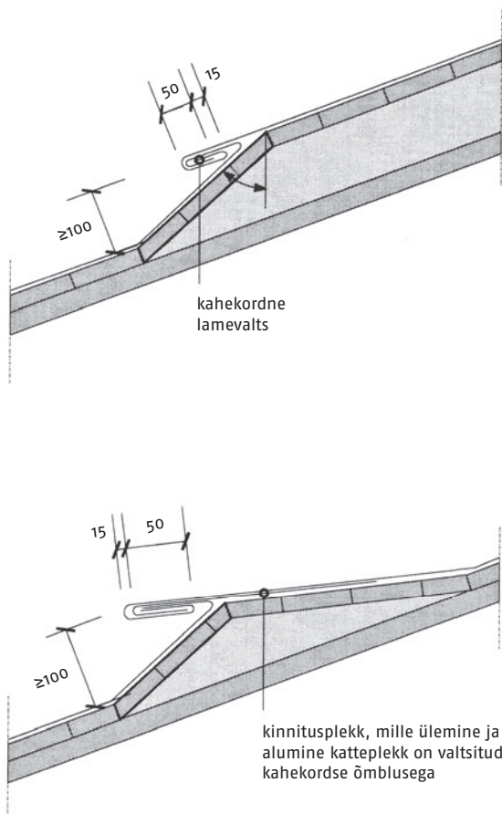
Joon. 15 Liikuvad õmblused. Mastaap 1:10
