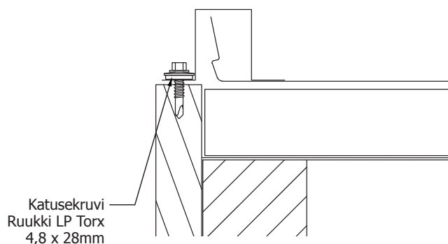
Joonis 4. Tugipleki positsioon räästas
