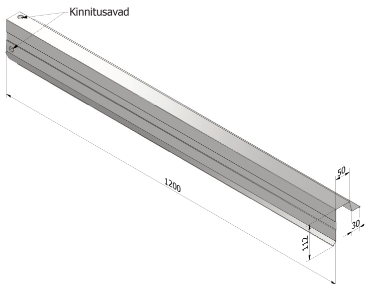
Joonis 3. Tugipleki kinnitamine
