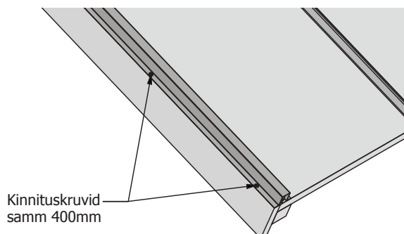
Joonis 3. Tugipleki kinnitamine
