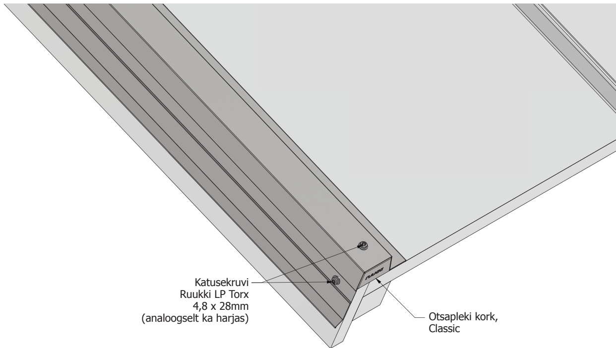
Joonis 5. Otsaplekkide paigaldus
