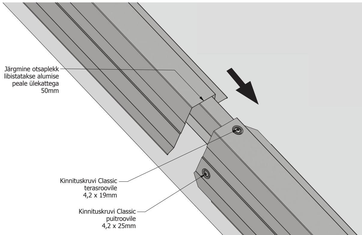
Joonis 6. Otsaplekkide paigaldus
