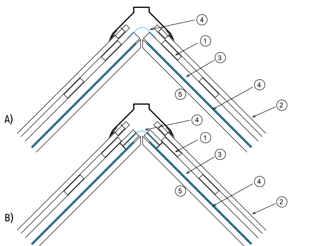
PULTOVÁ STŘECHA PŘÍČNÝ ŘEZ
