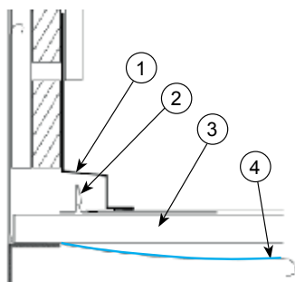
PŘECHOD STŘECHA – STĚNA, PŘÍČNÝ ŘEZ
