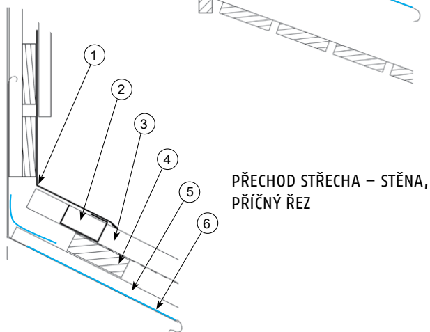
PŘECHOD STŘECHA – STĚNA, PŘÍČNÝ ŘEZ
