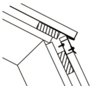
Příklad použití okapového lemování pro krytinu Classic u mansardové střechy.
