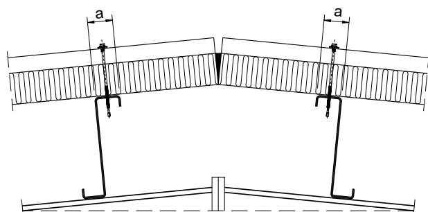
Rys. nr 21. Podpory skrajne a \geq 40 mm.
