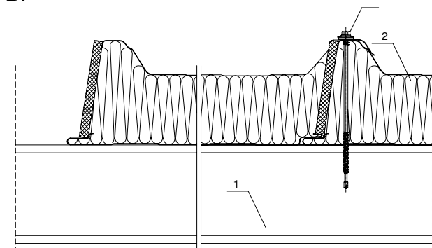
Rys. nr 19. Przykładowy montaż płyty, gdzie:
